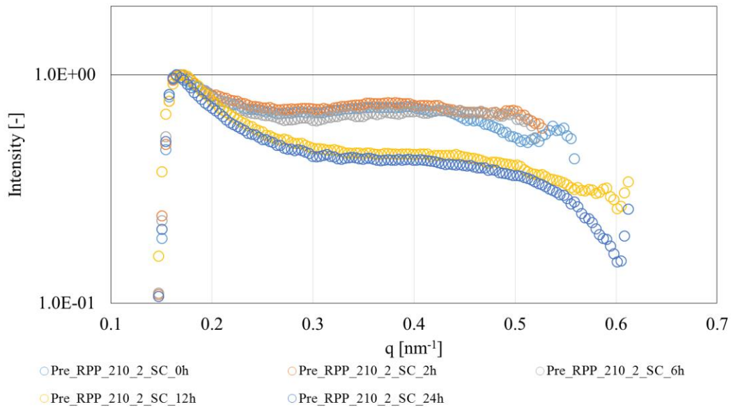
Fig.3 SAXS 分析結果(Pre-RP210°C2 分徐冷条件(SC))
