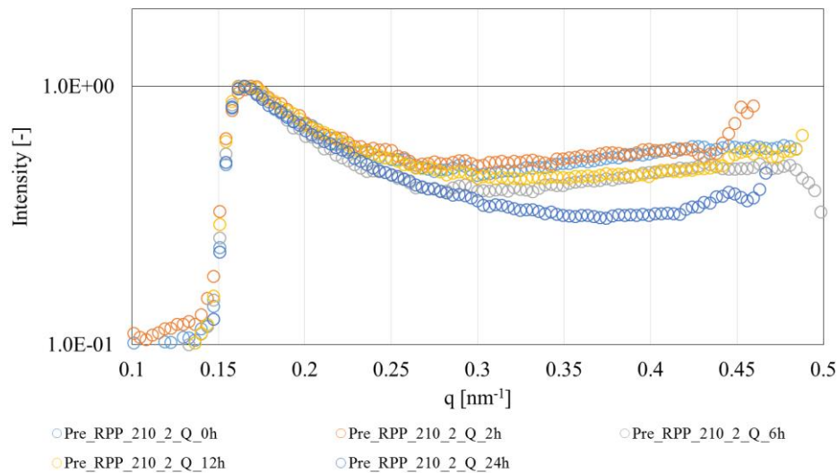
Fig.4 SAXS 分析結果(Pre-RP210°C2 分急冷条件(Q))
