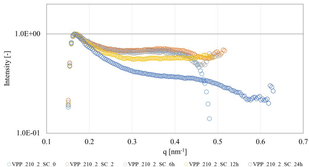
Fig.2 SAXS 分析結果 (VPP 210°C 2 分徐冷条件 (SC))
