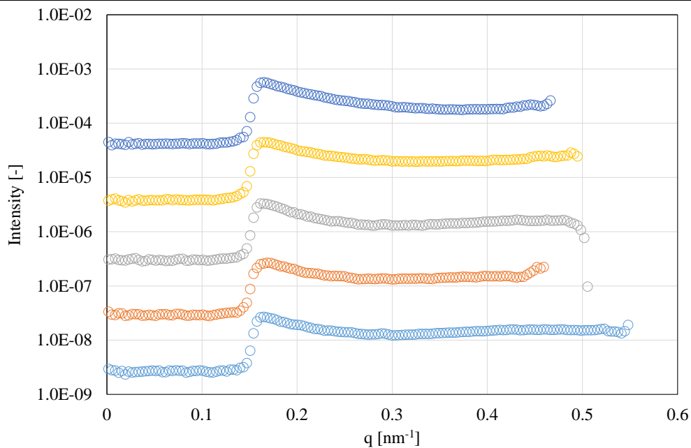
Fig.2-1 SAXS 分析結果(Pre-RPPP210°C2分急冷条件(Q), カメラ長 : ~1000mm)
