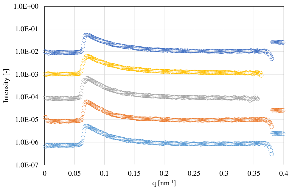
Fig.2-2 SAXS 分析結果(Pre-RPPP210°C2分急冷条件(Q), カメラ長 : ~2500mm)
