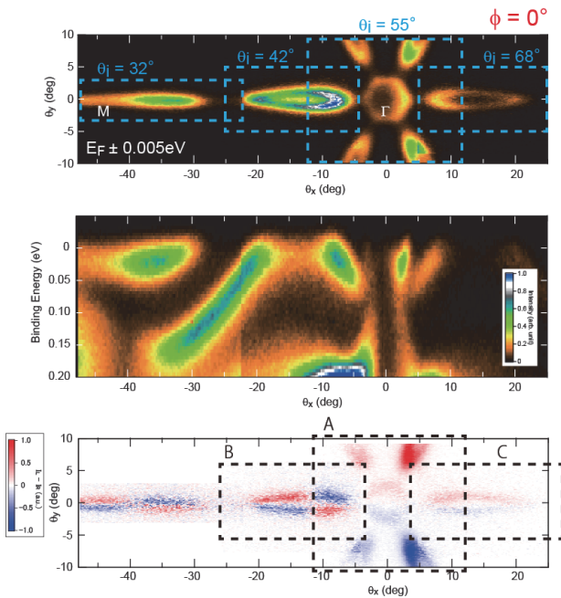
図2. Si(111)上のBi(111)単結晶薄膜の表面電子状態の円2色ARPESマッピング
