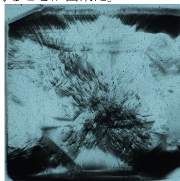
図2 絶縁HPHT基板上にエピ成長した結晶のX線トポグラフィ像 [-40-4]
