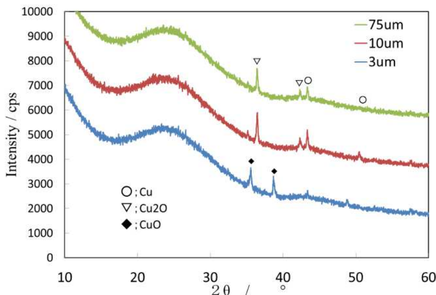
図4 X線回折測定結果.
