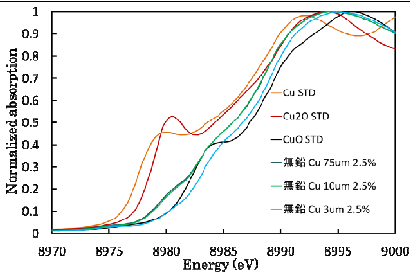
図5 銅緑無鉛上絵の XAFS(XANES)測定結果.
