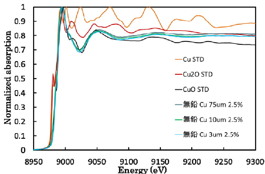
図6 銅緑無鉛上絵 XAFS(EXAFS)測定結果.
