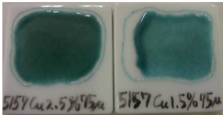
図2 添加量の変化による銅上絵の発色変化.
