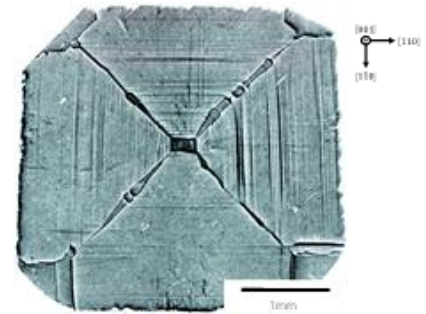
図2 X線トポグラフィ撮影像
