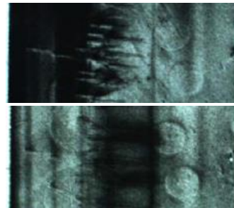
図2 HPHT基板（3mm角）のX線トポグラフィ像
