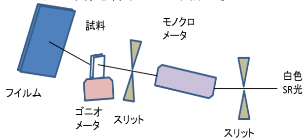
図1 X線トポグラフィの計測図
