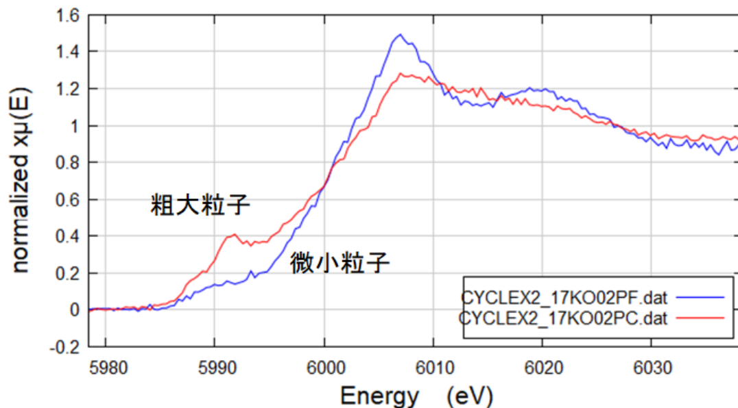
図 3. 神奈川においてサイクロンにより採取された微小側および粗大側の大気粒子試料の Cr K XANES スペクトル。青：微小粒子、赤：粗大粒子。
