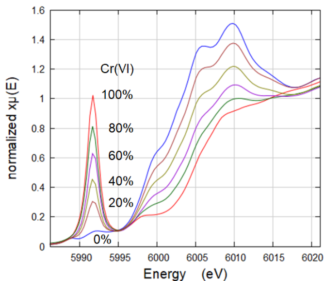
図 1. \text{Na}_2\text{CrO}_4 \cdot 4\text{H}_2\text{O} と \text{Cr}_2\text{O}_3 の混合試料の割合を 20% ずつ変化させたときの Cr K XANES スペクトルの変化
