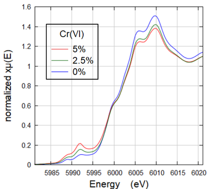
図 2. \text{Na}_2\text{CrO}_4 \cdot 4\text{H}_2\text{O} の含有割合の差が僅かであるときの Cr K XANES スペクトルのピーク高さの変化
