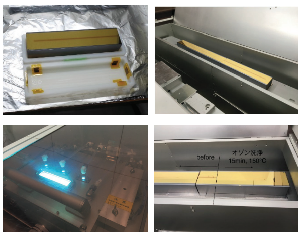
図2. Xeランプによる前置集光鏡のアッシング。
