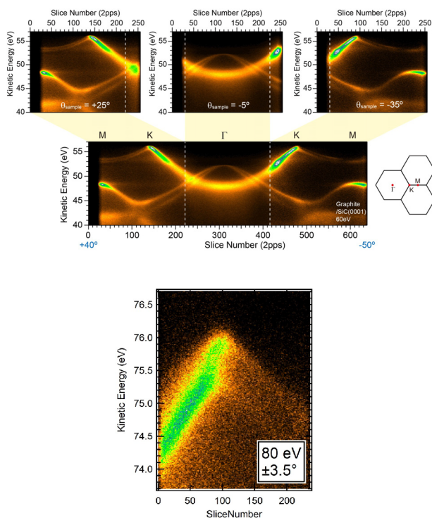
図3. 広範囲取り込みモードおよび高角度分解能モードでの、単結晶グラファイトの角度分解光電子スペクトル。
