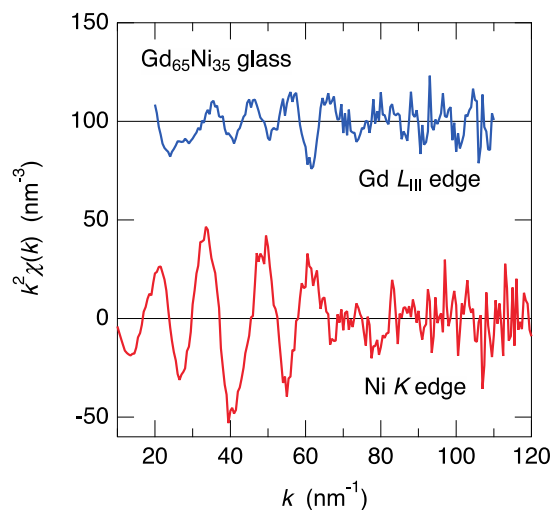
図1：よくアニールされたGd 65 Co 35 金属ガラスのGd L III およびCo K吸収端付近で得られた k^2\chi(k) スペクトル。
