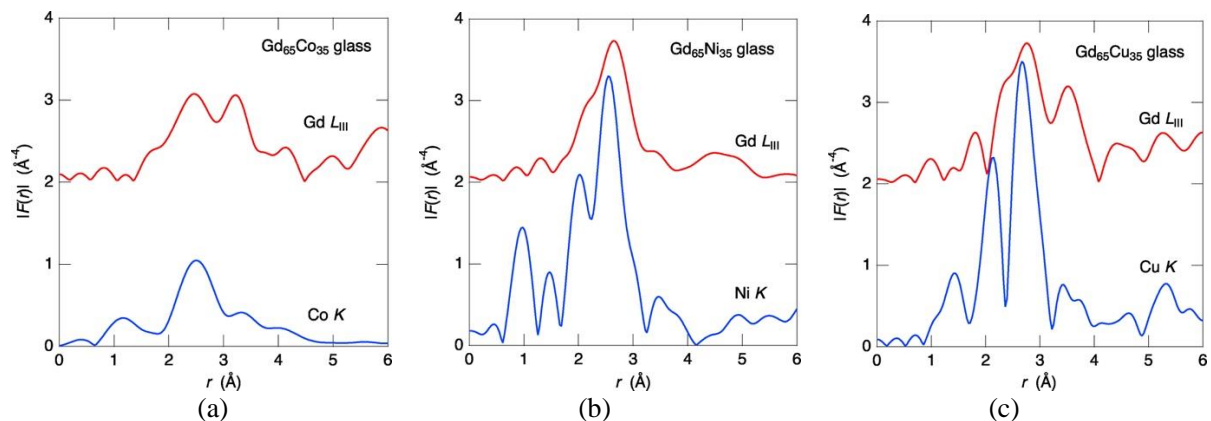
図1:十分にアニールされた(a) Gd 65 Co 35 、(b) Gd 65 Ni 35 および(c) Gd 65 Cu 35 の k^3\chi(k) のフーリエ変換 |F(r)| 。上: Gd L III 、下: TM K吸収端付近の結果。
