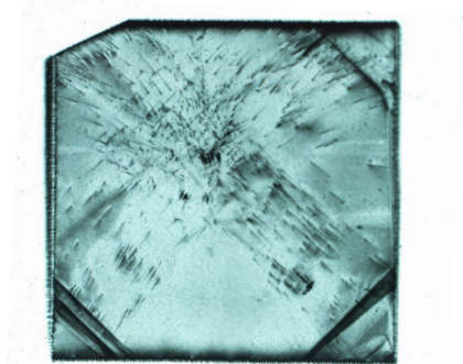
図2 HPHT基板（3mm角）のX線トポグラフィ像 [044]
