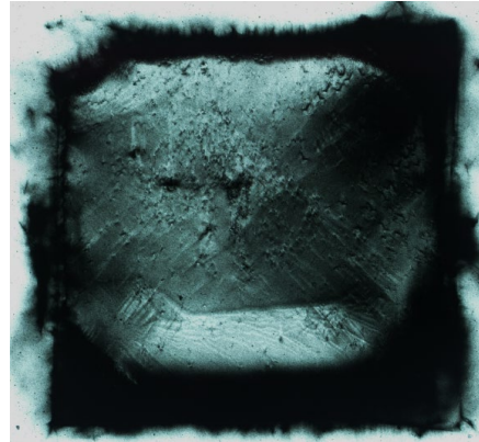
図2 エピタキシャル成長膜（3mm角）のX線トポグラフィ像 [404]
