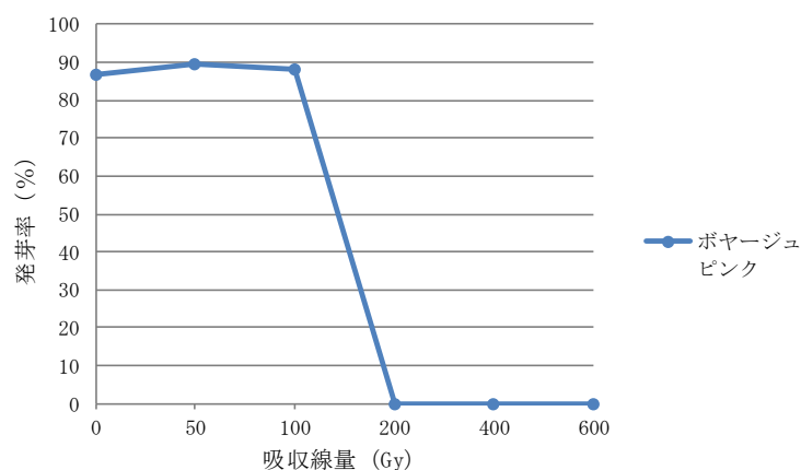
図1 シンクロトロン光を照射したトルコギキョウ種子「ボヤージュピンク」の播種60日後の発芽率
