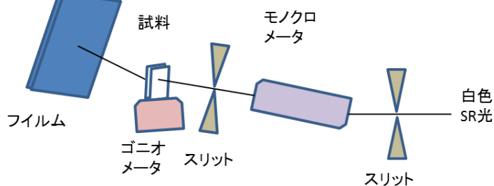
図1 X線トポグラフィの計測図
