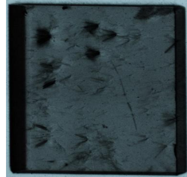
図2 CVD基板（3mm角）の X線トポグラフィ像
