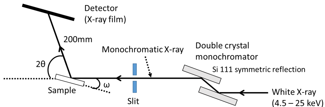
図1 透過 Laue 配置による X 線トポグラフィー測定
