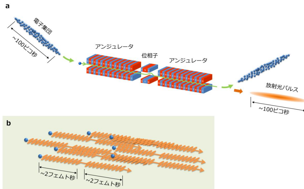
図 1: アンジュレータによる放射光発生の様式図。放射光パルスの時間幅は電子集団の空間広がりによって決まる (a)。放射光パルスには個々の電子が放射した多数の短い波 (波束) が含まれている。本研究では二台のアンジュレータを並べて 10 回だけ振動する長さ 2 フェムト秒の波束のペアを生成した (b)。波束ペアの時間間隔は二台のアンジュレータの間にある位相子電磁石で電子の軌道を蛇行させて調整する。
