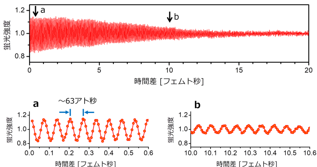
図 2 : 上段 : 波束ペアの時間間隔を変えながら測定したキセノン原子の内殻空孔状態からの蛍光強度。下段 : 時間領域 a、b 付近の拡大図。二つの波束による量子状態の干渉効果のため、63 アト秒周期の変動が観測される。波束ペアの時間間隔が大きくなると内殻空孔状態の電子緩和のために周期変動の振幅が減衰する。
